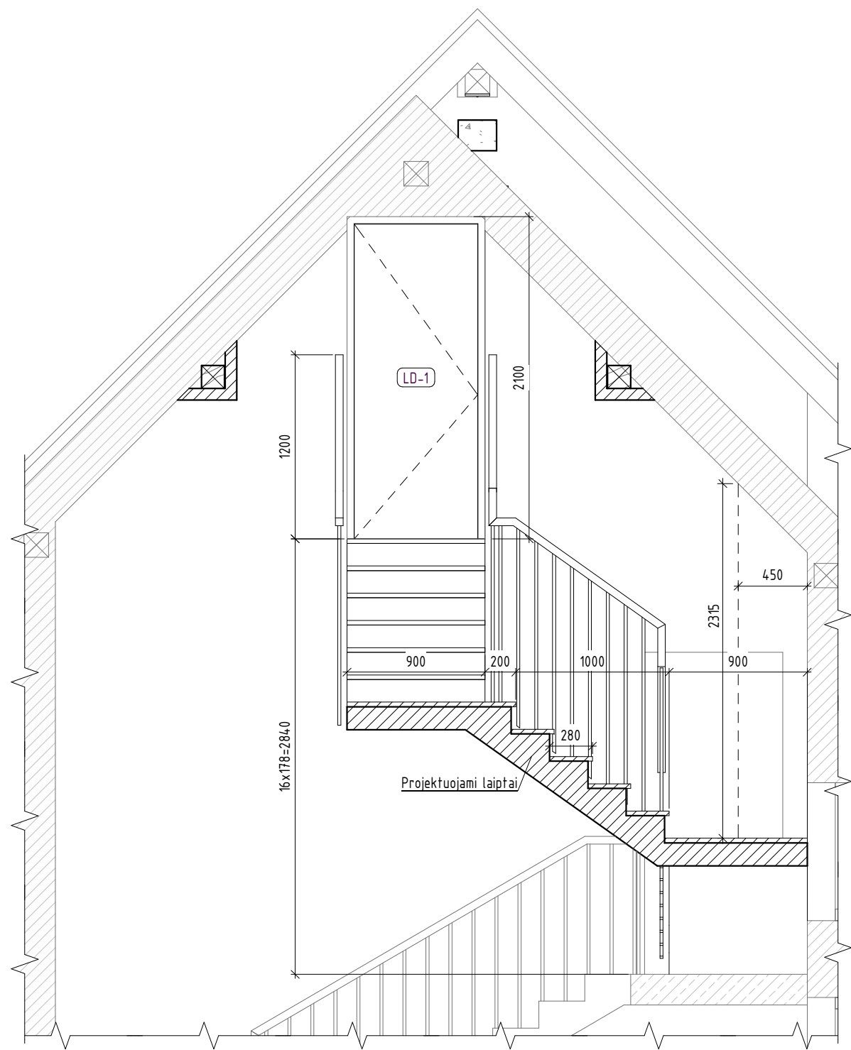
PJŪVIS 1-1 (1 : 35)
