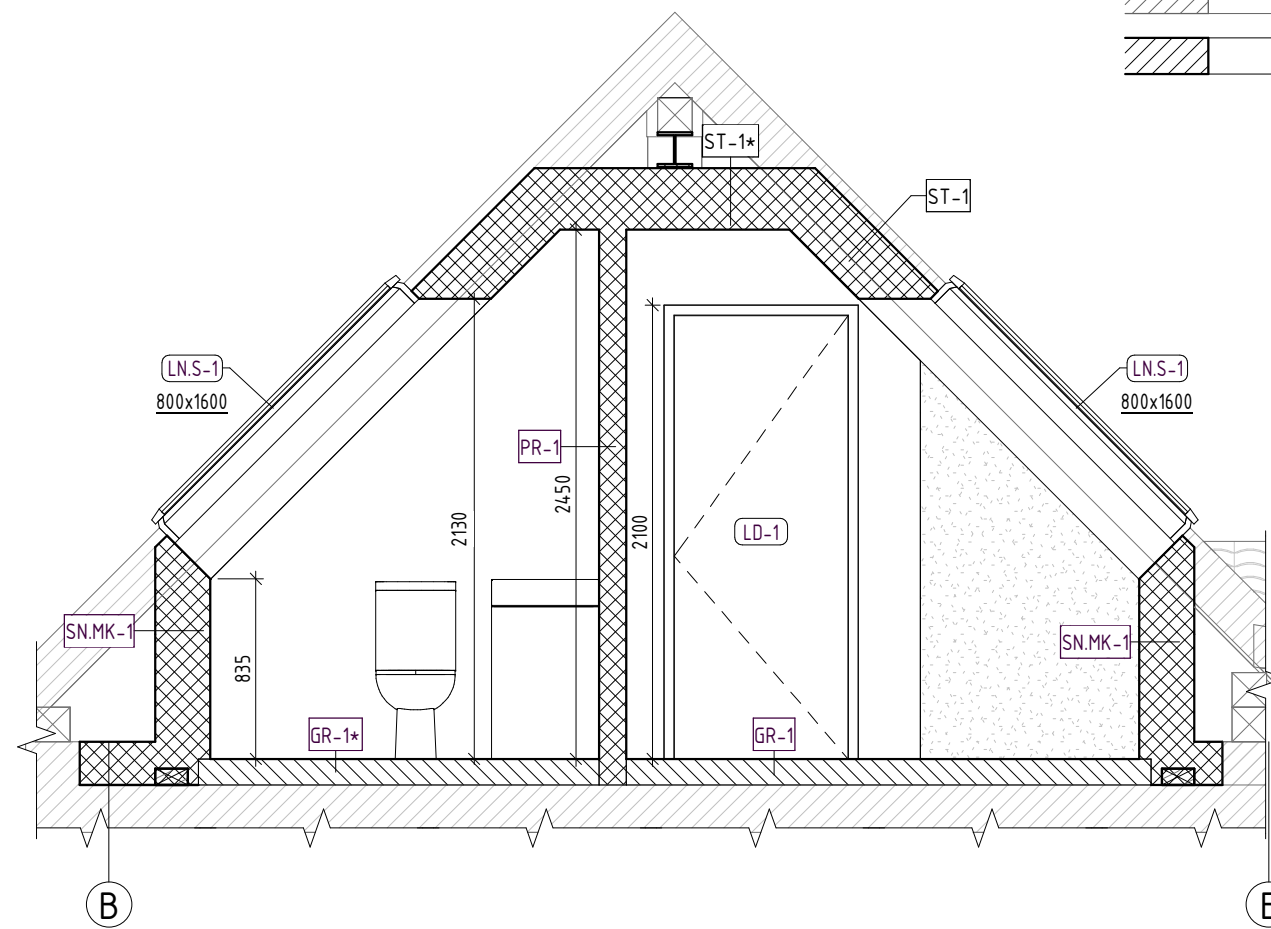
PJŪVIS 2-2 (1 : 35)
